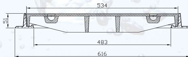
SECCION A-A
