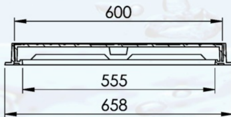
SECCIÓN B-B
