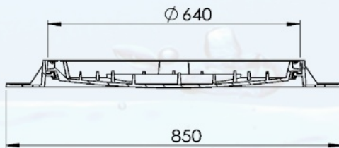
SECCIÓN B-B ESCALA 1 : 10
